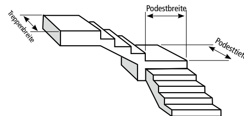
5. Treppe 90° abgewinkelt mit Podest
