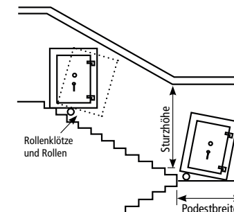
6. Treppe 180° abgewinkelt mit Podest
