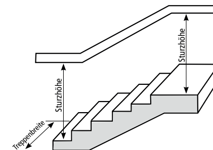
2. gerade Treppe mit Unterzug
